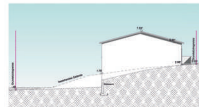
Ansicht West
