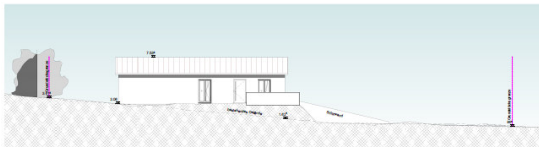
Ansicht Süd
