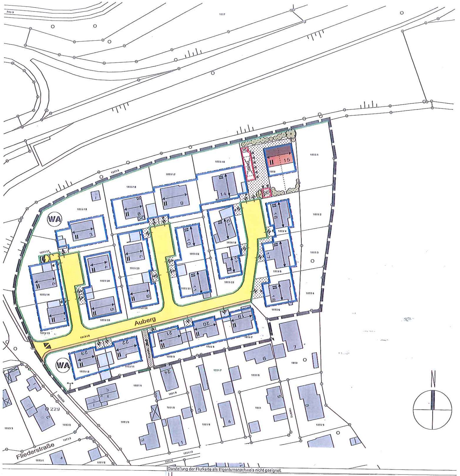
Lageplan zum Bebauungsplan mit Grünordnungsplan Tiefenbach - Siedlung - Erweiterung Deckblatt 01
